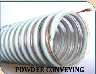
PU HOSE WITH RIGID HELIX Serie 3PUR M - AL - ANT
